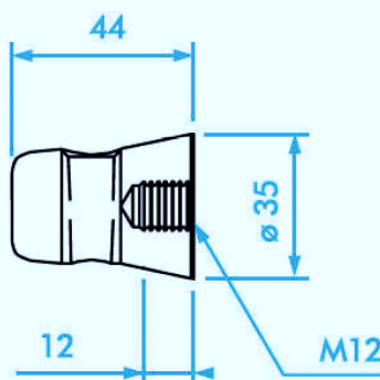
WKC Mezzo Spinotto acciaio Half conical coupler
