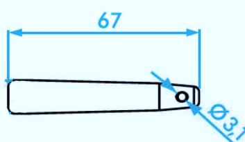
WKC Spina conica acciaio Spigot steel
