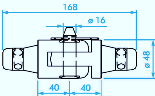
STW Snodo per torre elevazione Hinge for Tower Truss
