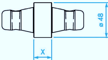
WKCX Spinotto con distanza X Conical coupler Spacers
